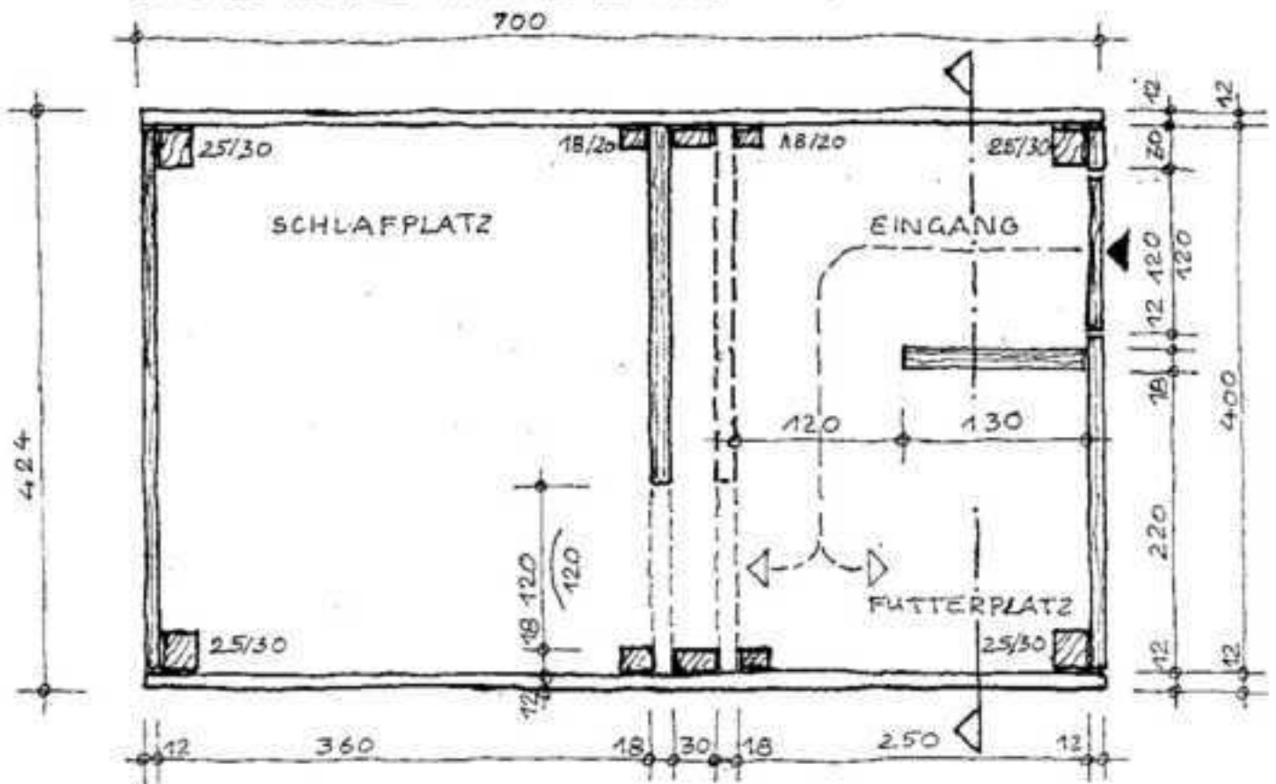
GRUNDRISS
