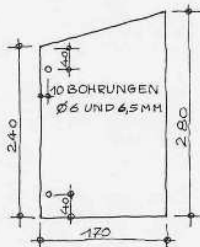
SEITENWÄNDE 2x
