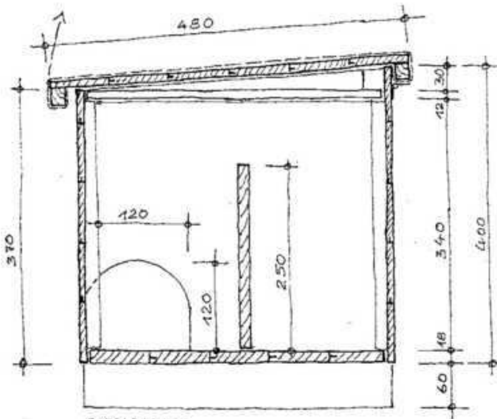
SCHNITT
